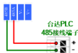
台达PLC连接EG20
